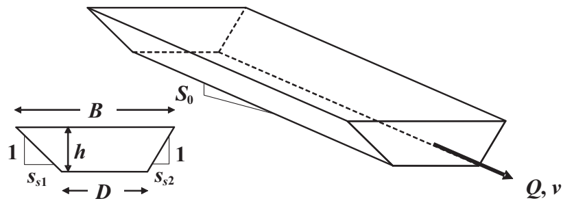
Rys. 6.4 Ilustracja koryta trapezoidalnego zastępującego w module programowym QUAL2K koryto naturalne (Chapra et al. 2007)
